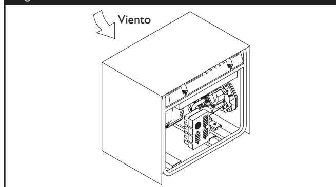
Figura 32 — Clima Frío Estructura de Protección
